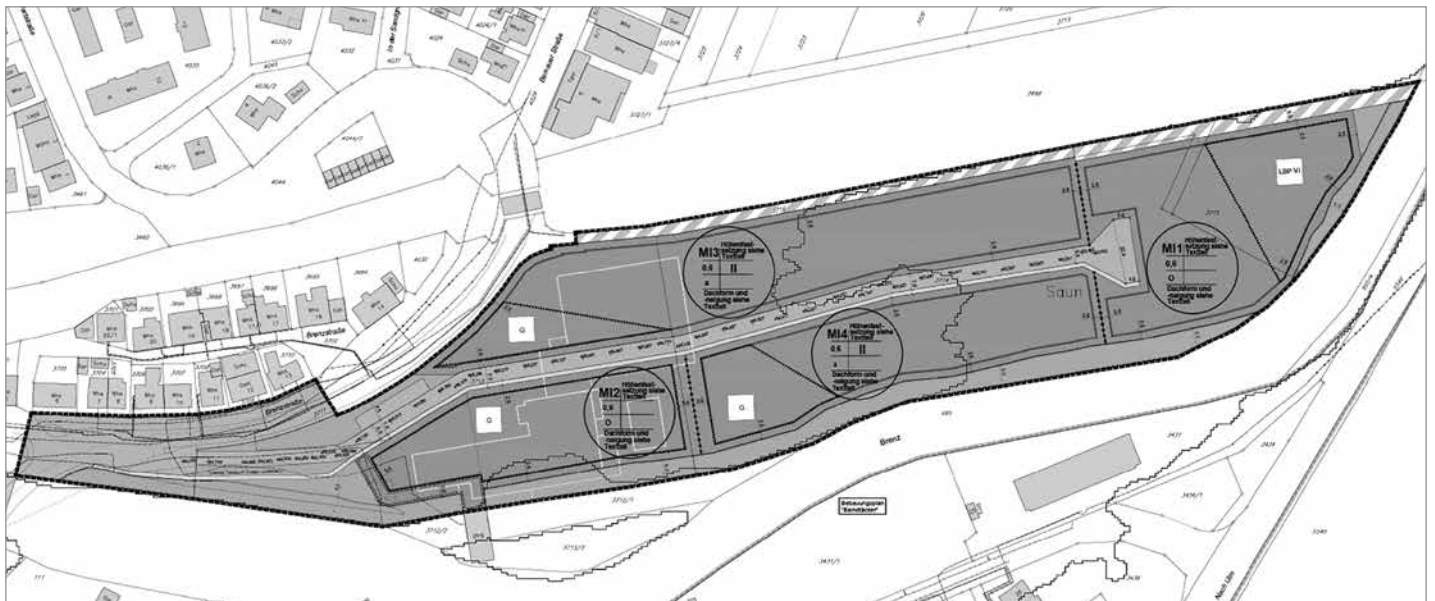
Ausschnitt Bebauungsplan „Liegelind-Areal“ vom 30.06.2022, unmaßstäblich, genordet
